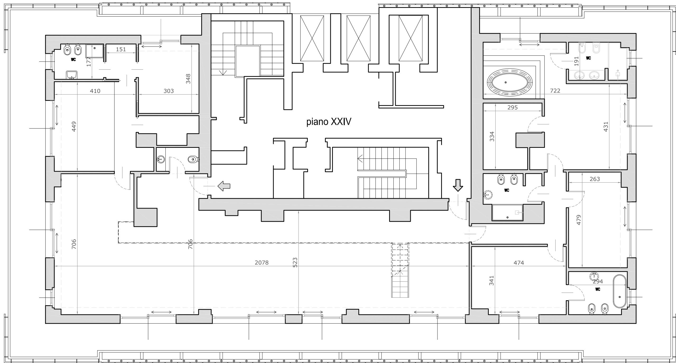
PIANTA PIANO VENTiquATTRESIMO SCALA 1:100 SITUAZIONE ATTUALE
